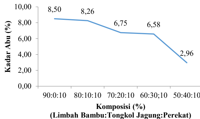
Gambar 2. Grafik kandungan Abu Briket Limbah Bambu dan Janggel Jagung
