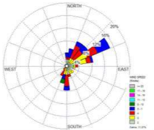
Gambar 13. Mawar angin untuk titik K dekat Tarakan
