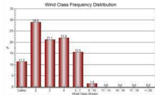
Gambar 14. Distribusi frekuensi kemunculan kecepatan angin di dekat Tarakan
